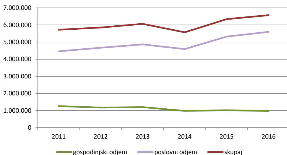
Grafikon 20: Poraba zemeljskega plina v občini Škofja Loka v obdobju 2011 – 2016 v Sm 3
