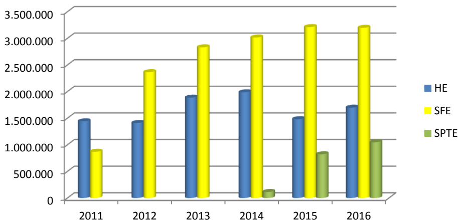
Grafikon 18: Razpršeni viri za proizvodnjo električne energije v občini Škofja Loka v obdobju 2011 – 2016 po inštalirani moči (kW) vir: Elektro Gorenjska d.d.
