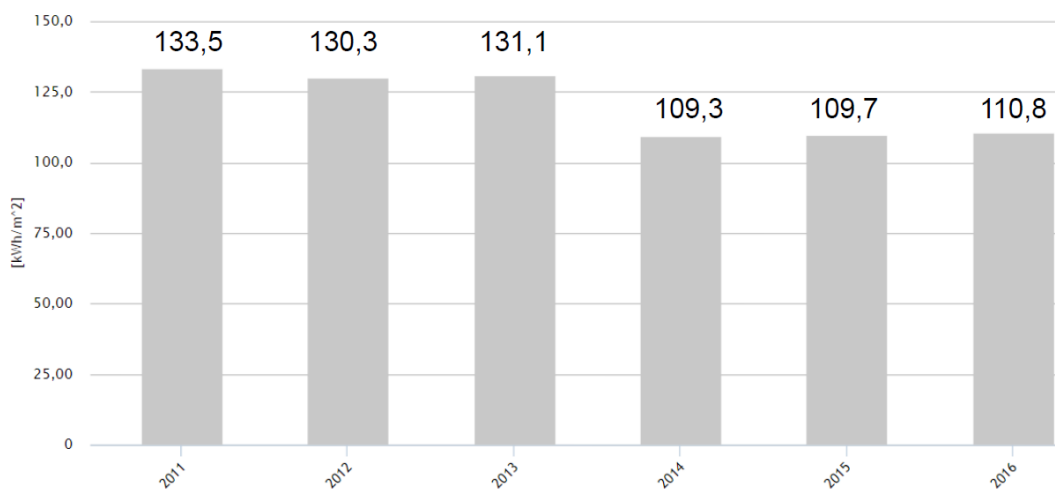
Grafikon 5: Gibanje specifične porabe energije v osnovni bilančni skupini v kWh/m 2 vir: ENEKOM, Inštitut za energetska svetovanj, d.o.o.
