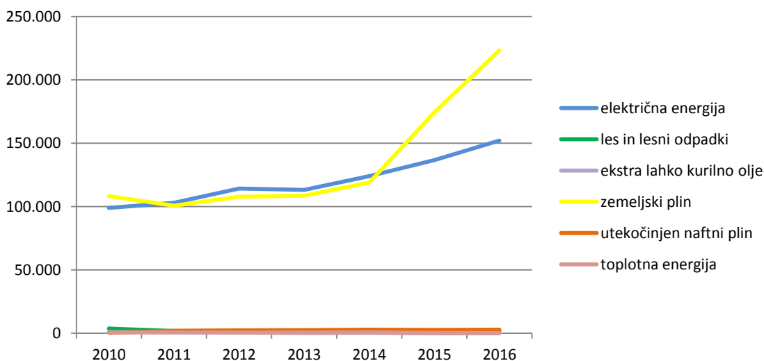
Grafikon 11: Raba energije v industriji v obdobju 2010 – 2016 v občini Škofja Loka (MWh)
