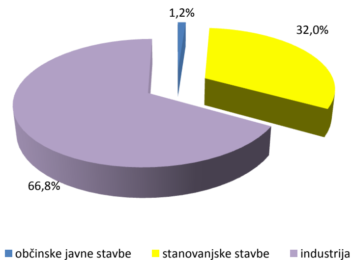
Grafikon 15: Raba toplotne energije po skupinah v občini Škofja Loka v letu 2016
