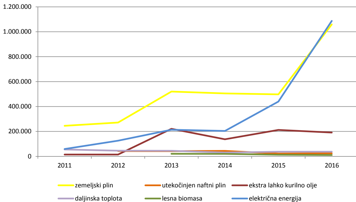
Grafikon 6: Raba toplotne in električne energije v občini Škofja Loka v skupini ostale stavbe v obdobju 2011 - 2016 vir: sistem spremljanja rabe energije (ENEKOM, Inštitut za energetska svetovanj, d.o.o.)
