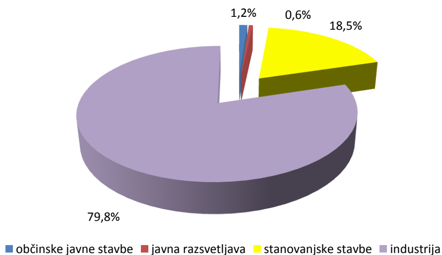
Grafikon 16: Rabe električne energije po skupinah v občini Škofja Loka v letu 2016
