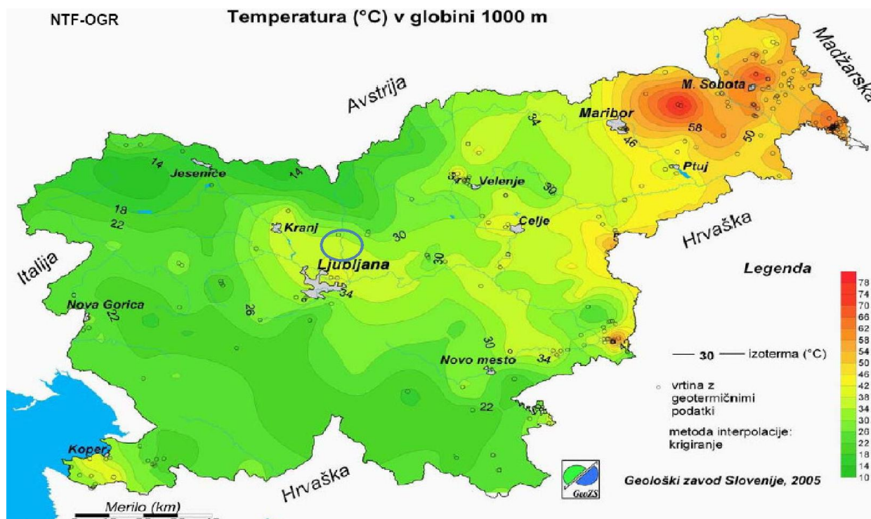
Karta 4: Geološka prognoza z energetskega izračuna vir: Geološki zavod Slovenije
