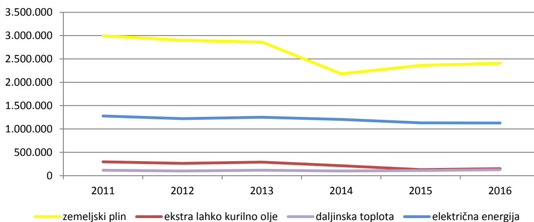
Grafikon 3: Raba toplotne in električne energije v občini Škofja Loka v občinskih javnih stavbah v osnovni bilančni skupini v obdobju 2011 - 2016
