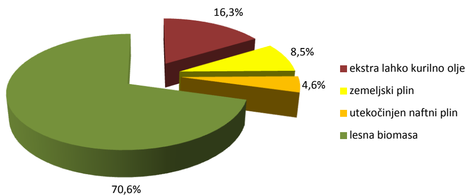
Grafikon 1: Poraba toplotne energije v občini Škofja Loka v stanovanjskem sektorju v letu 2016
