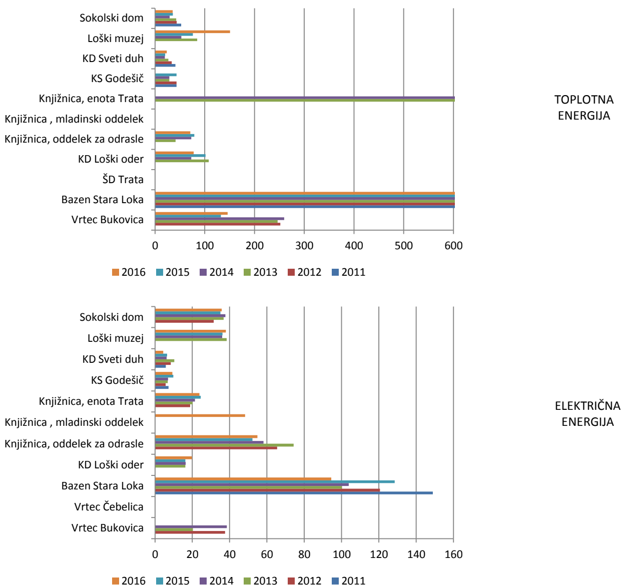
Grafikon 7: Specifična poraba energije(energijsko število) v skupini ostale stavbe v obdobju 2011 – 2016 v kWh/m 2 vir: sistem spremljanja rabe energije (ENEKOM, Inštitut za energetske svetovanj, d.o.o.)
