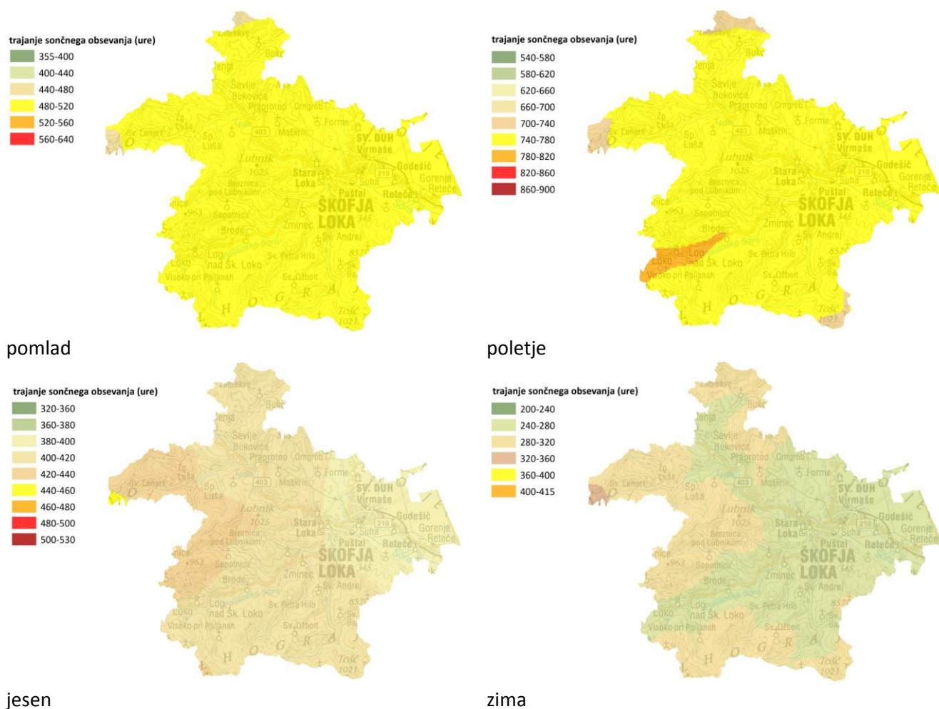
Karta 3: Povprečno trajanje sončnega obsevanja (ur) 1971 - 2000 v občini Škofja Loka
