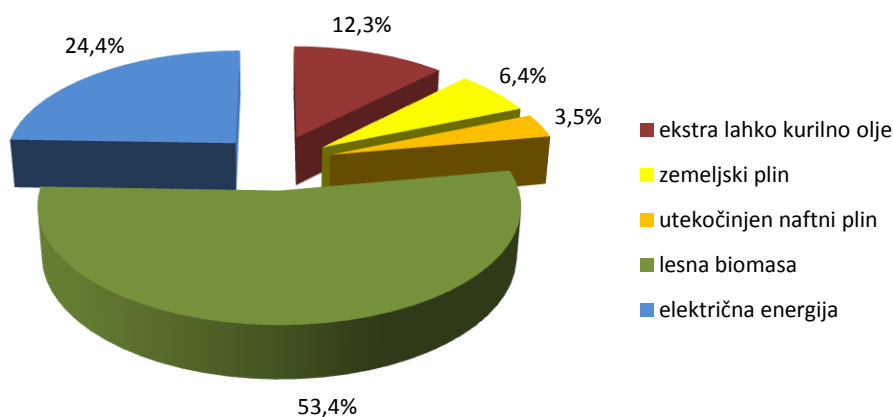
Grafikon 2: Skupna bilanca toplotne in električne energije v občini Škofja Loka v stanovanjskem sektorju v letu 2016
