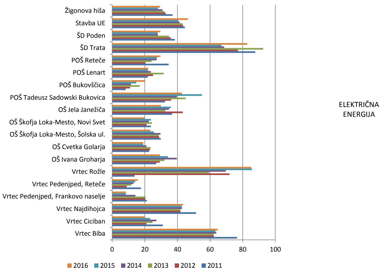
Grafikon 4: Specifična poraba energije (energijsko število) v osnovni bilančni skupini v obdobju 2011 – 2016 v kWh/m 2 vir: sistem spremljanja rabe energije (ENEKOM, Inštitut za energetske svetovanj, d.o.o.)
