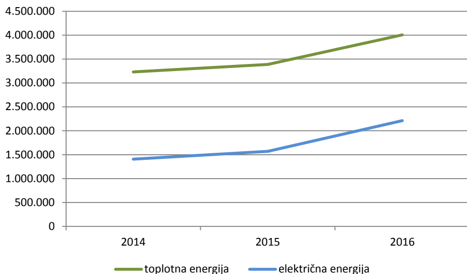
Grafikon 8: Raba toplotne in električne energije v občini Škofja Loka v občinskih javnih stavbah v letih 2014, 2015 in 2016
