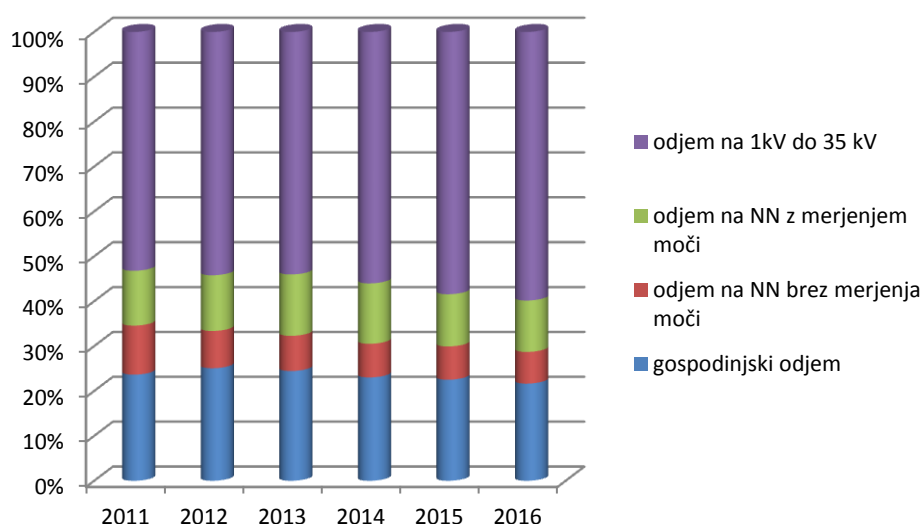
Grafikon 13: Raba električne energije v občini Škofja Loka v obdobju 2011 – 2016 (MWh) vir: Elektro Gorenjska d.d.
